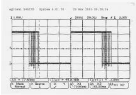
Génération d'un signal carré sous Linux chargé
